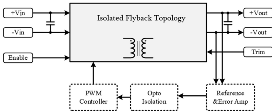
ESAS 单路电路图
