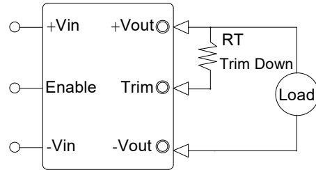
图 2. 电阻调整输出电压示意图(下调)
