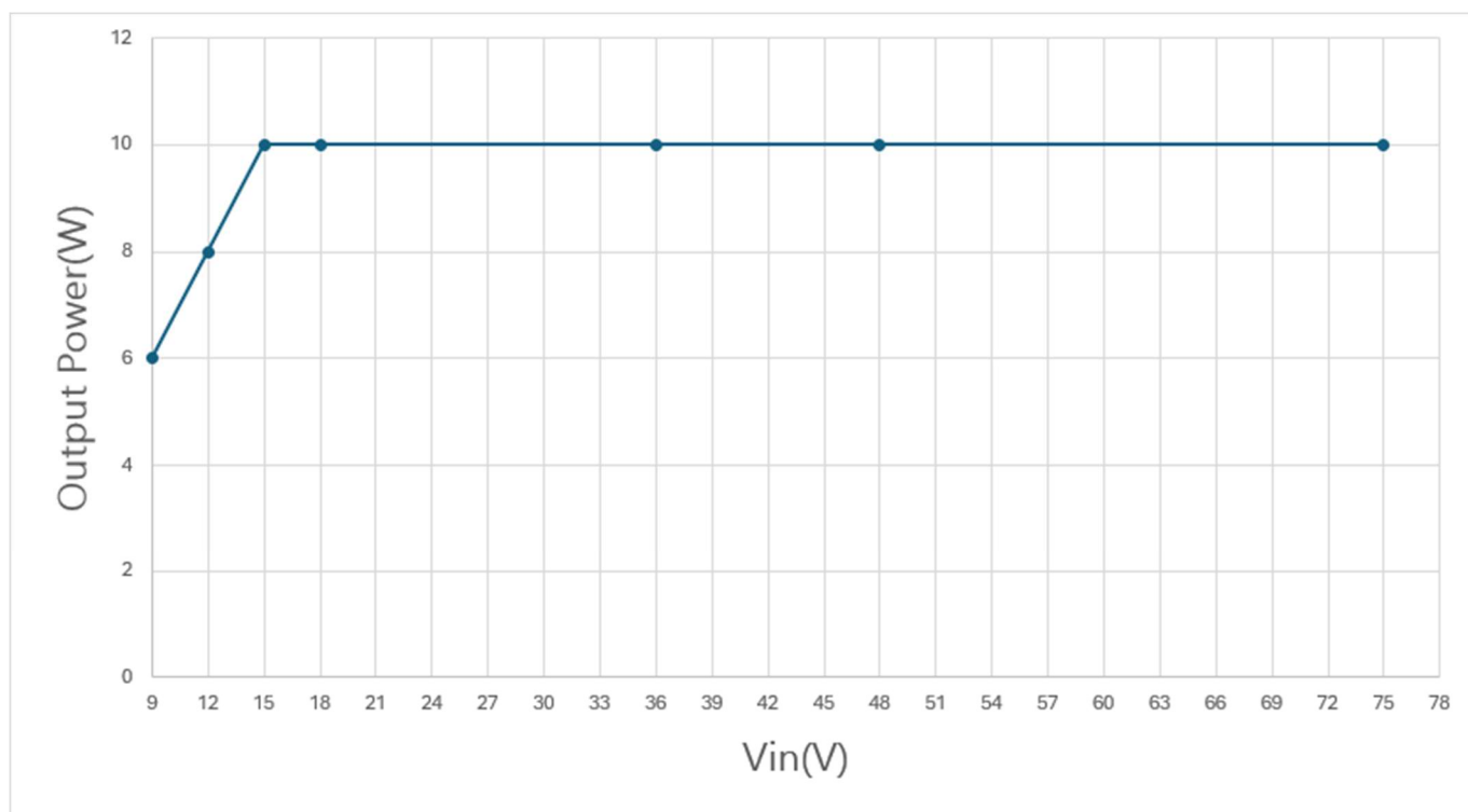
输出额定功率 VS 输入电压
