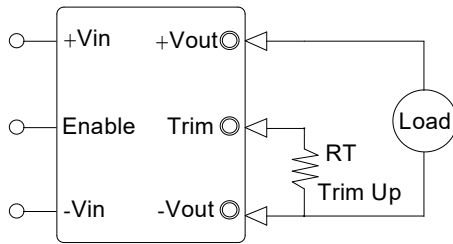
图 1. 电阻调整输出电压示意图(上调)
