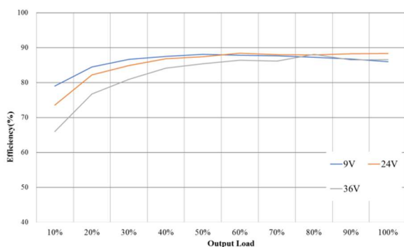
图 1: 效率值 VS 输出负载 分别于最小、额定、最大输出电压时
