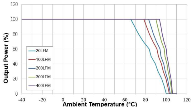
图 3 : 环境温度 VS 输出效率额降曲线
