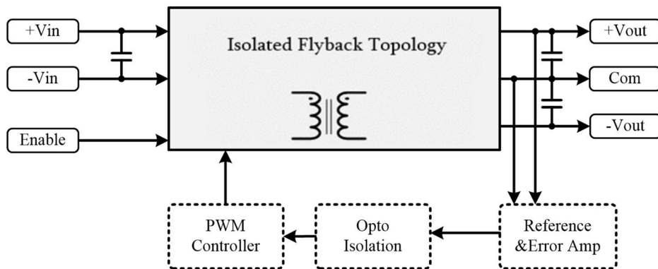
ESAS 正负双路电路图
